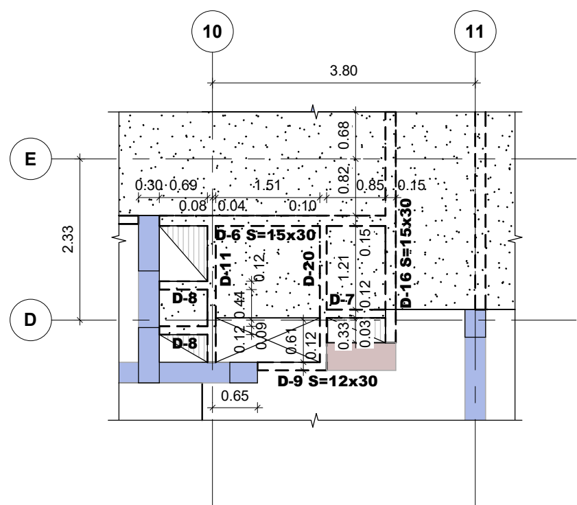
DETALLE PLACA ADICIONAL PISO 14 Y PISO 15 Escala 1 : 75
